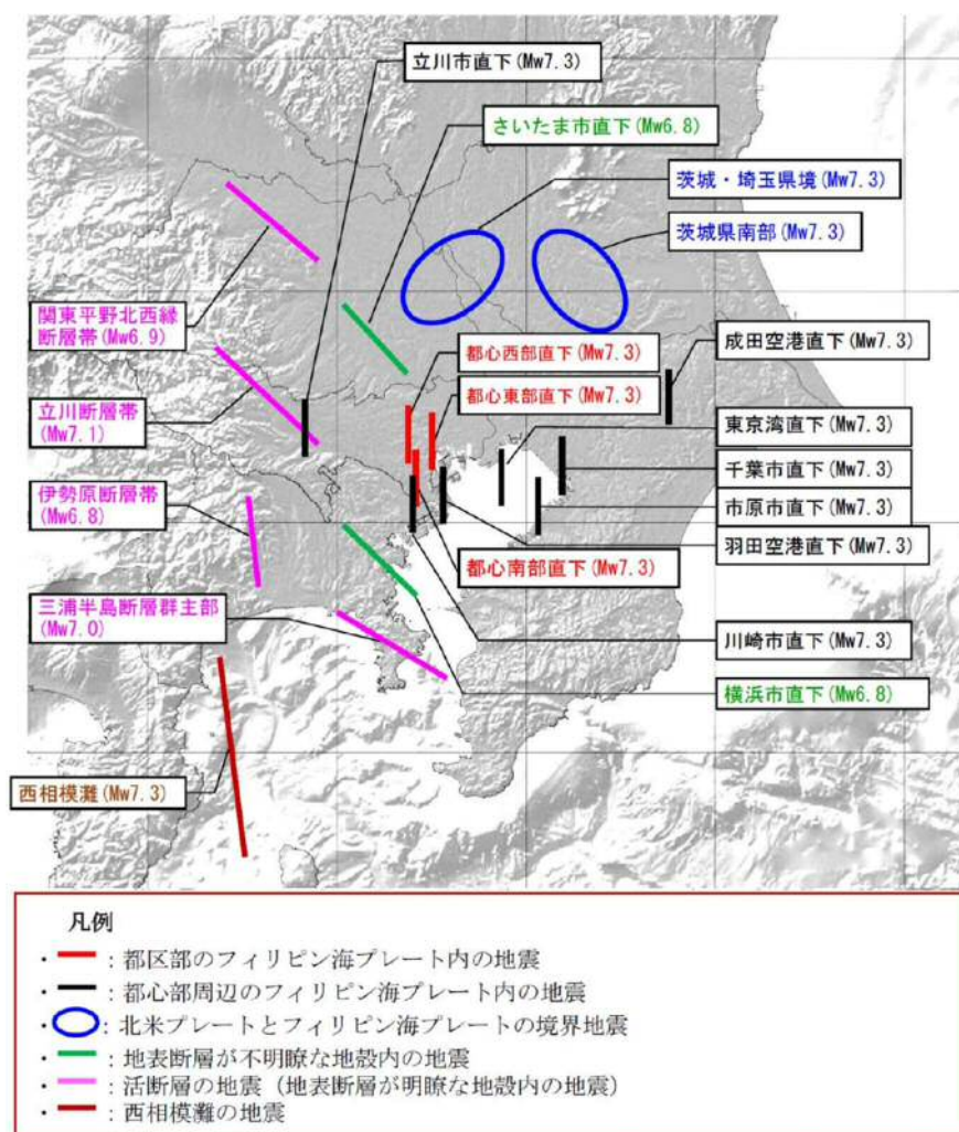
図 M7 クラスの首都直下地震の断層位置 内閣府(2013)
